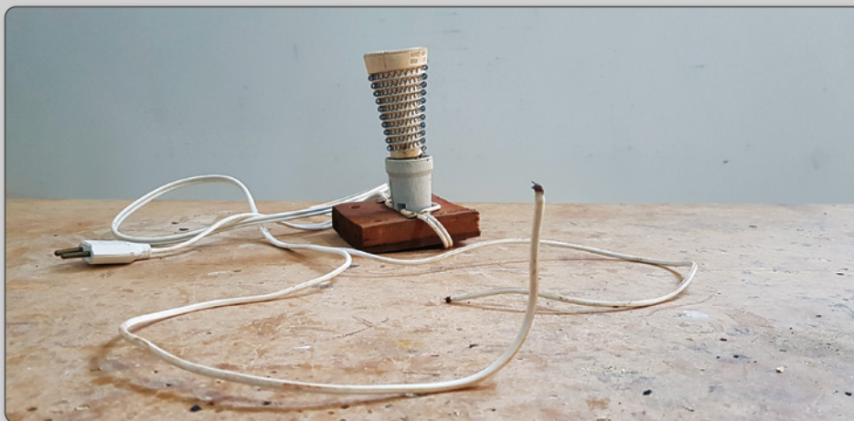
Figura 15 – Incrustador elétrico de cera com resistência cônica
